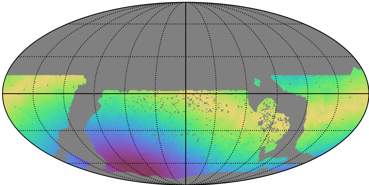
extra_ss_neo7_v3.4_10yrs WFD g band: Max moonDistance
