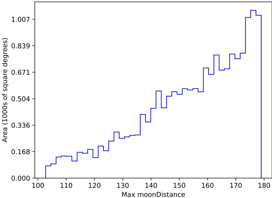
extra_ss_neo7_v3.4_10yrs WFD g band: Max moonDistance
