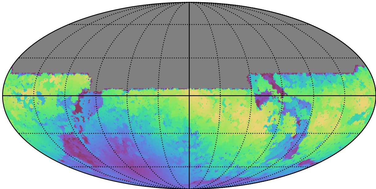
extra_ss_neo7_v3.4_10yrs All sky y band: Max moonDistance
