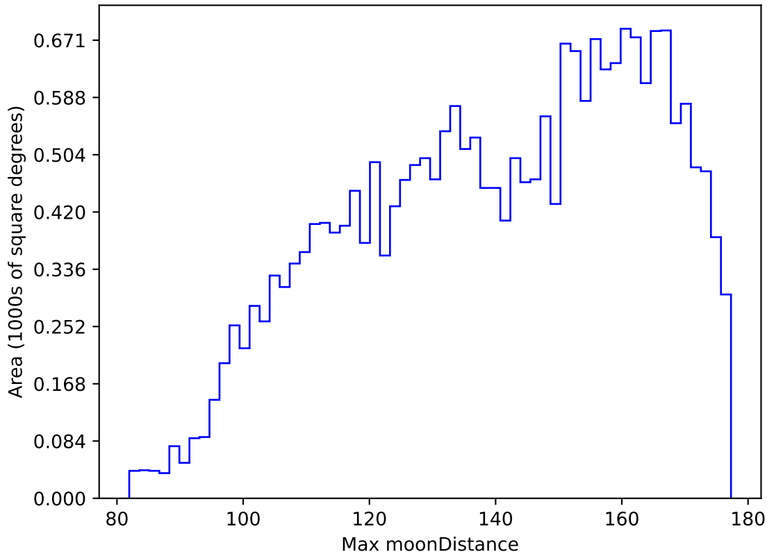
extra_ss_neo7_v3.4_10yrs All sky y band: Max moonDistance
