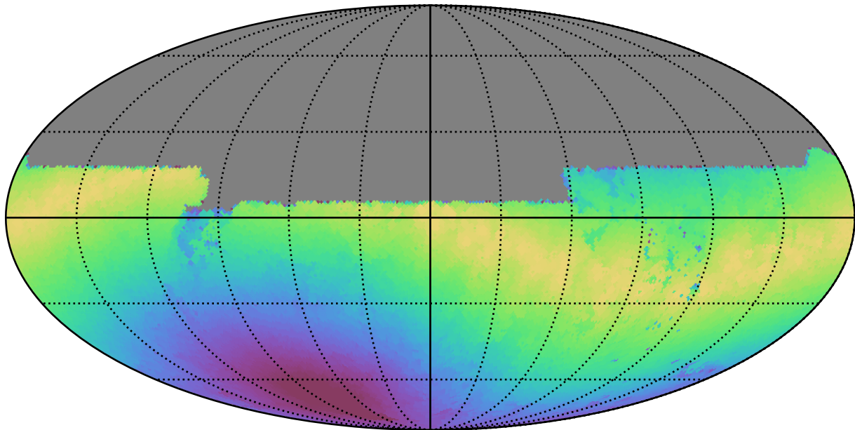
extra_ss_neo7_v3.4_10yrs All sky u band: Max moonDistance
