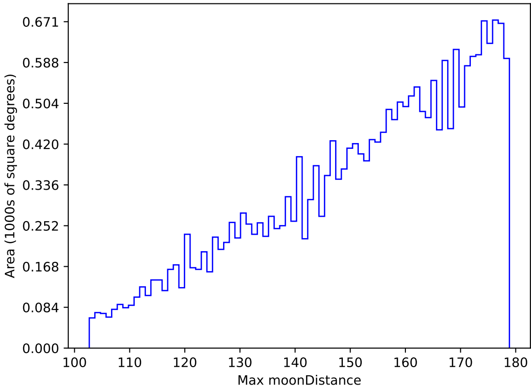
extra_ss_neo7_v3.4_10yrs All sky u band: Max moonDistance
