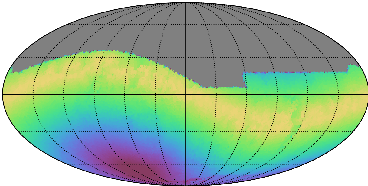
extra_ss_neo7_v3.4_10yrs All sky r band: Max moonDistance
