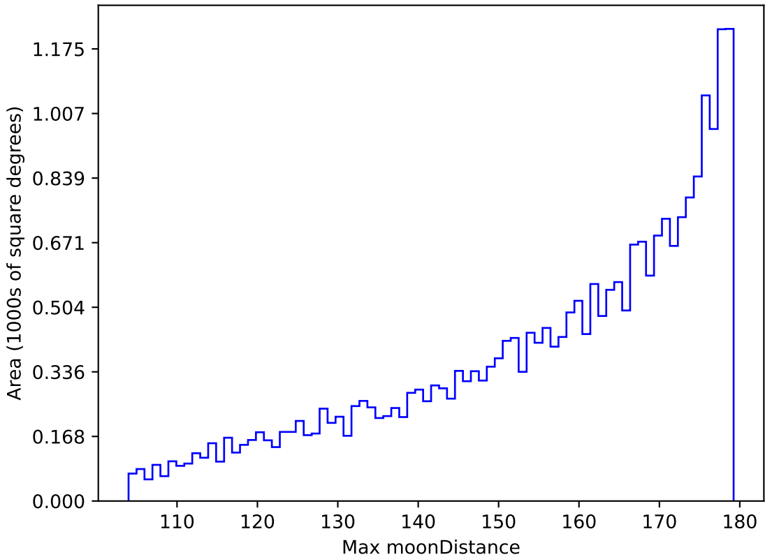
extra_ss_neo7_v3.4_10yrs All sky r band: Max moonDistance
