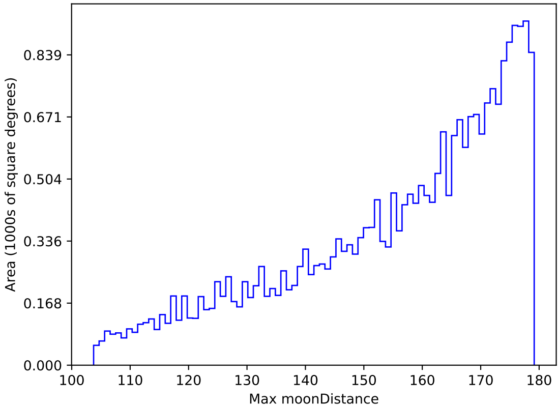
extra_ss_neo7_v3.4_10yrs All sky i band: Max moonDistance
