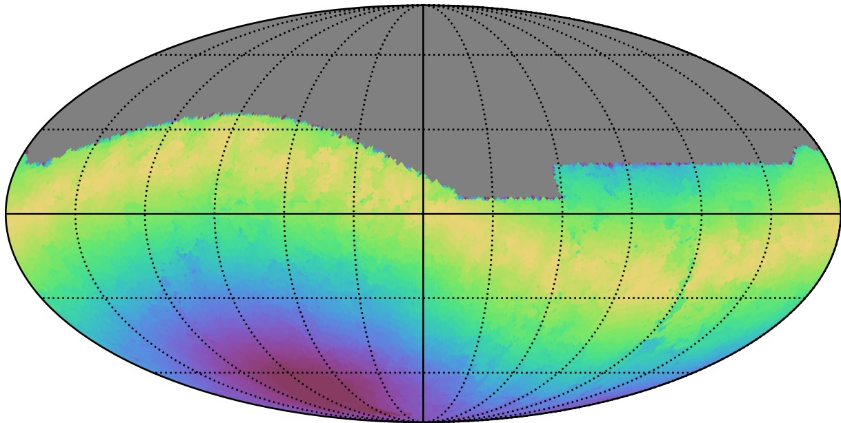
extra_ss_neo7_v3.4_10yrs All sky g band: Max moonDistance
