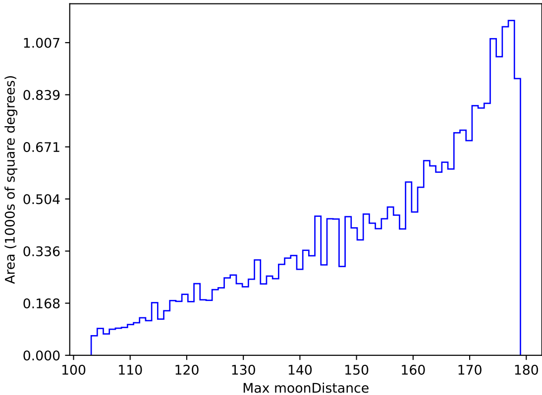
extra_ss_neo7_v3.4_10yrs All sky g band: Max moonDistance
