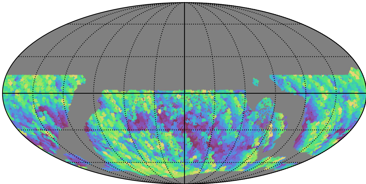
extra_ss_neo7_v3.4_10yrs WFD y band: Max airmass
