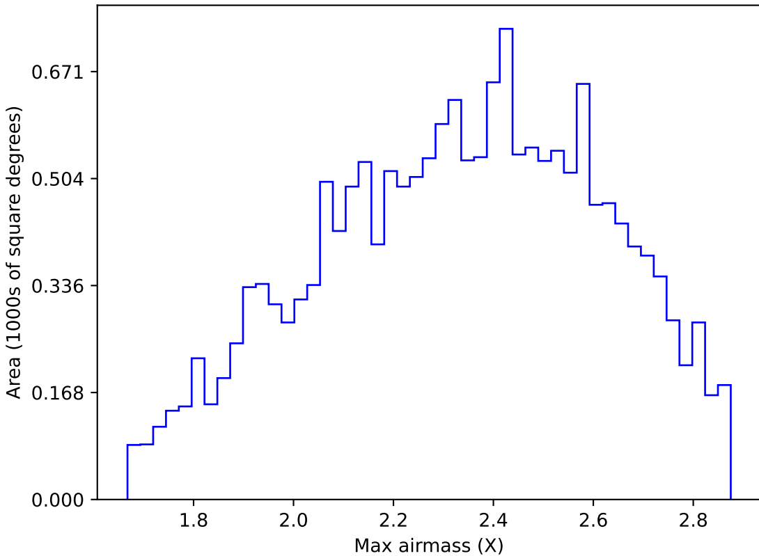
extra_ss_neo7_v3.4_10yrs WFD y band: Max airmass
