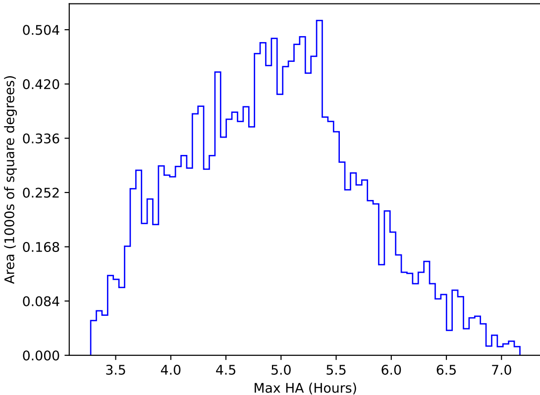
extra_ss_neo7_v3.4_10yrs WFD z band: Max HA
