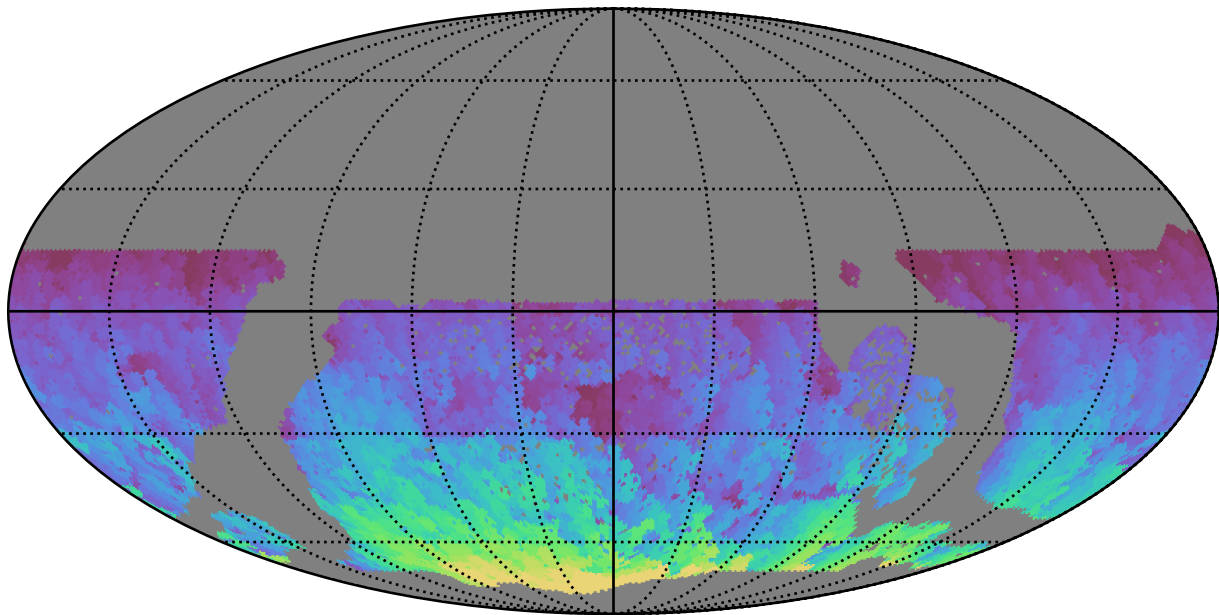
extra_ss_neo7_v3.4_10yrs WFD y band: Max HA
