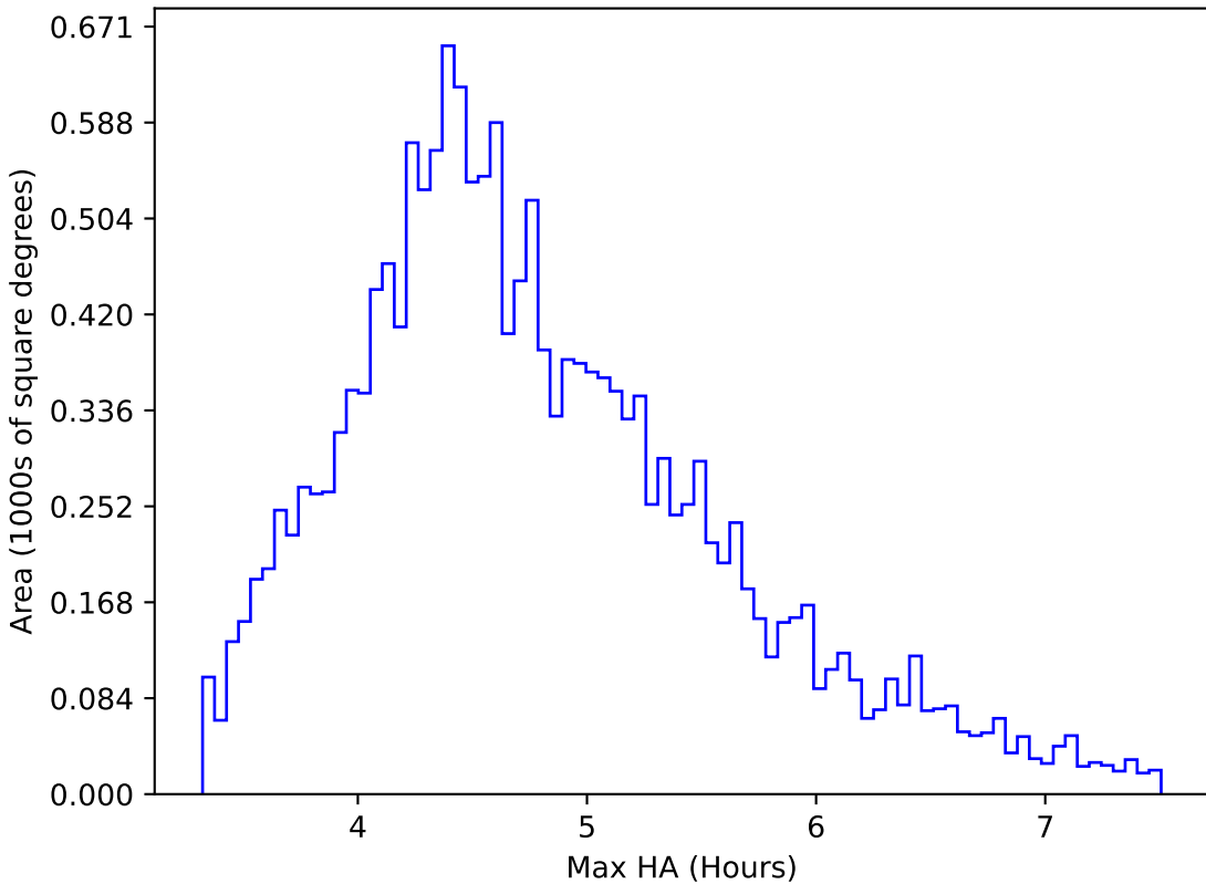
extra_ss_neo7_v3.4_10yrs WFD y band: Max HA
