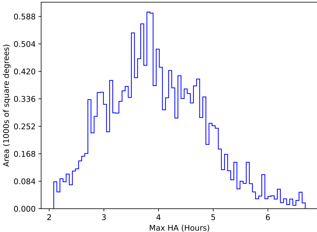
extra_ss_neo7_v3.4_10yrs WFD u band: Max HA
