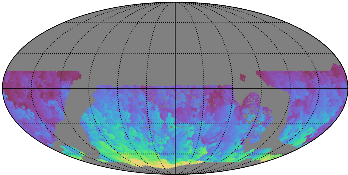
extra_ss_neo7_v3.4_10yrs WFD r band: Max HA
