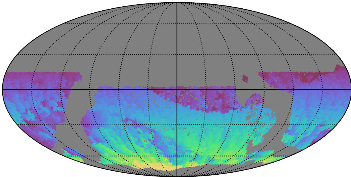
extra_ss_neo7_v3.4_10yrs WFD i band: Max HA
