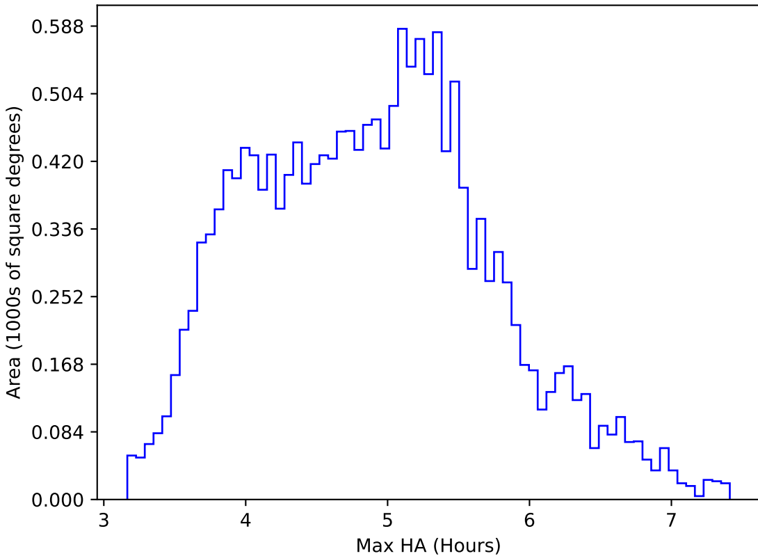
extra_ss_neo7_v3.4_10yrs WFD i band: Max HA
