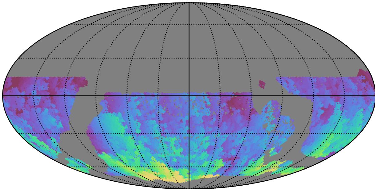
extra_ss_neo7_v3.4_10yrs WFD g band: Max HA
