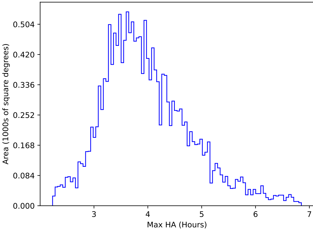
extra_ss_neo7_v3.4_10yrs WFD g band: Max HA
