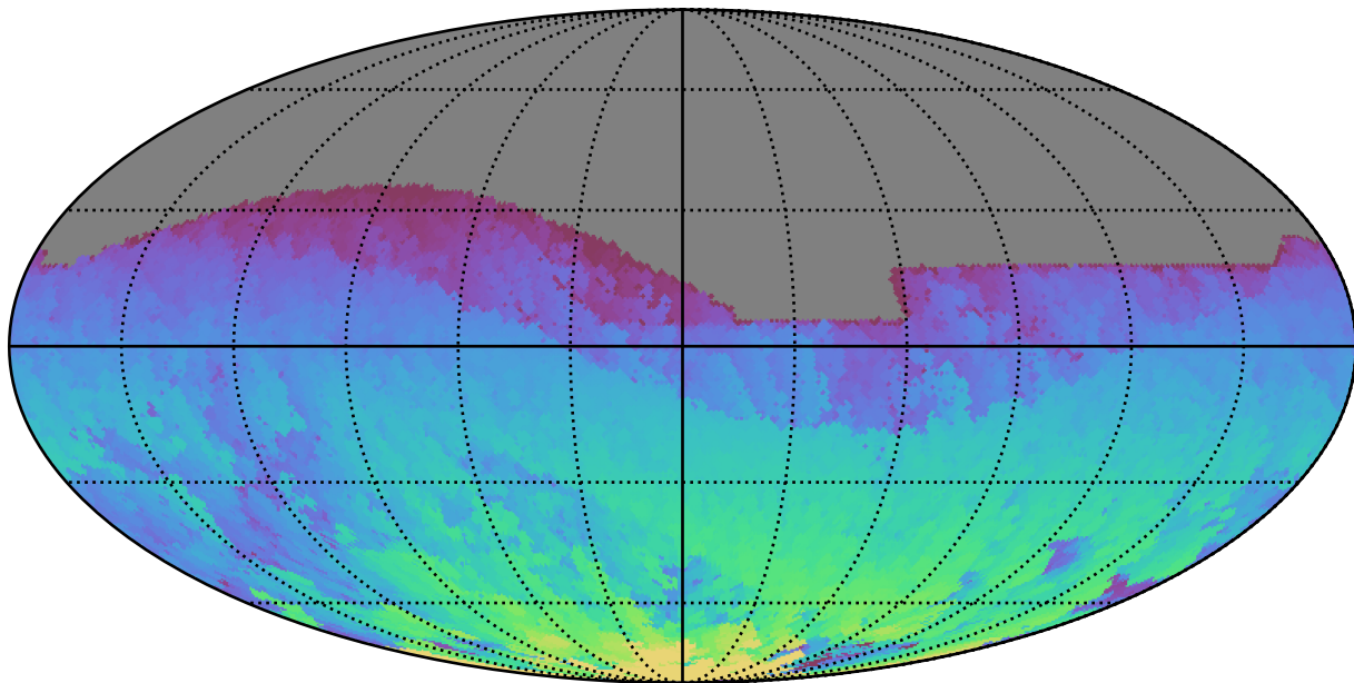
extra_ss_neo7_v3.4_10yrs All sky z band: Max HA
