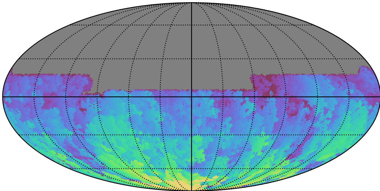
extra_ss_neo7_v3.4_10yrs All sky u band: Max HA
