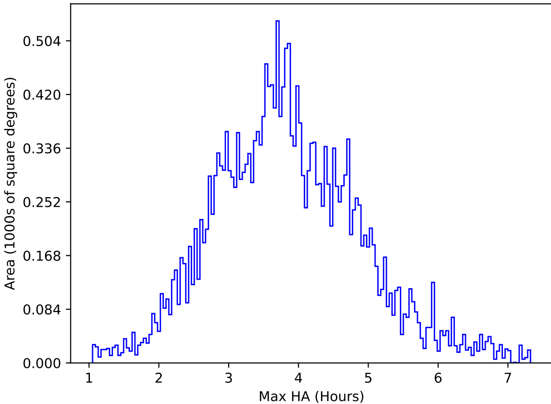
extra_ss_neo7_v3.4_10yrs All sky u band: Max HA
