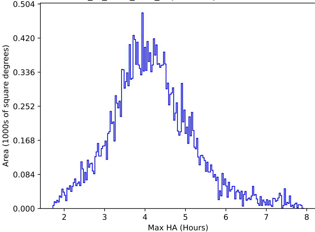
extra_ss_neo7_v3.4_10yrs All sky r band: Max HA
