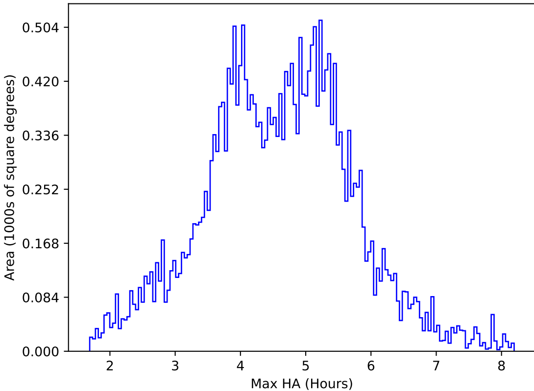
extra_ss_neo7_v3.4_10yrs All sky i band: Max HA
