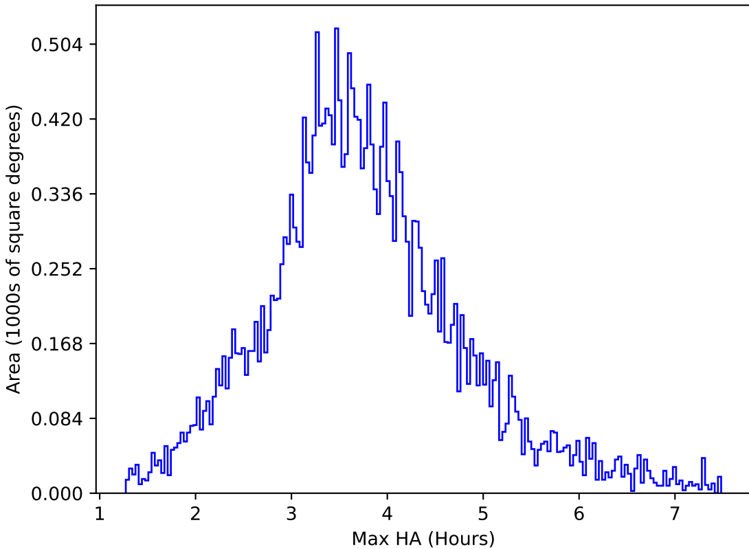
extra_ss_neo7_v3.4_10yrs All sky g band: Max HA
