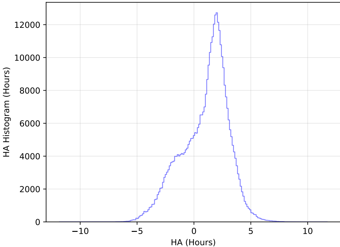
extra_ss_neo7_v3.4_10yrs WFD y band: HA Histogram
