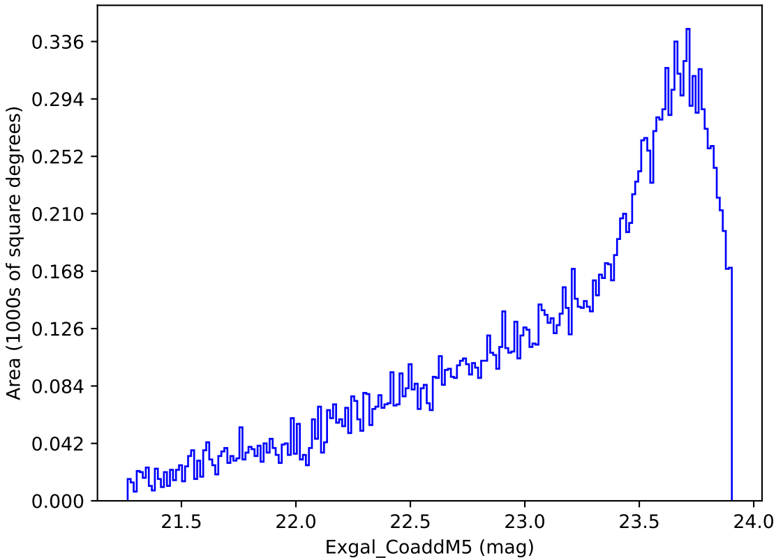
extra_ss_neo7_v3.4_10yrs Yr 3-4 y band: Exgal_CoaddM5
