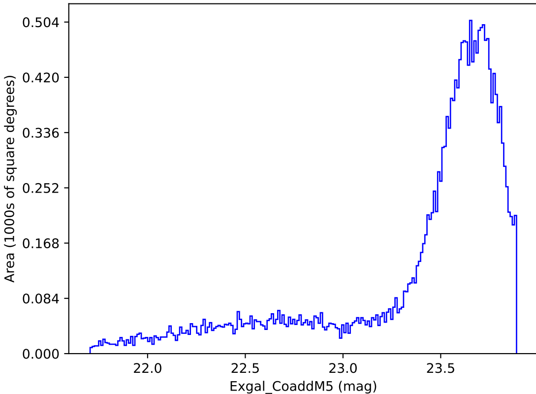
extra_ss_neo7_v3.4_10yrs Yr 1 y band: Exgal_CoaddM5
