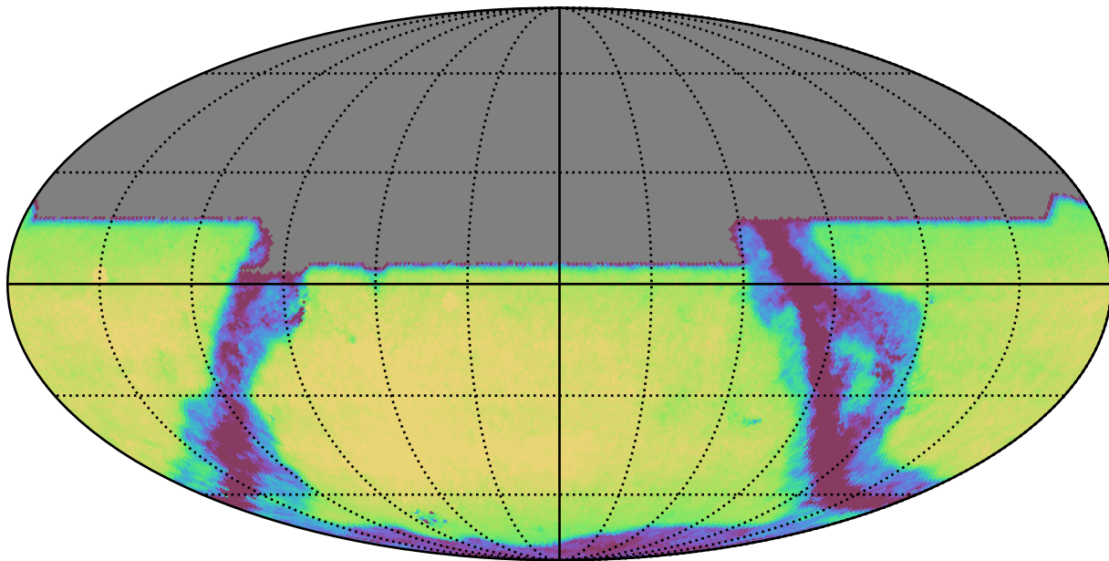
extra_ss_neo7_v3.4_10yrs All sky y band: Exgal_CoaddM5
