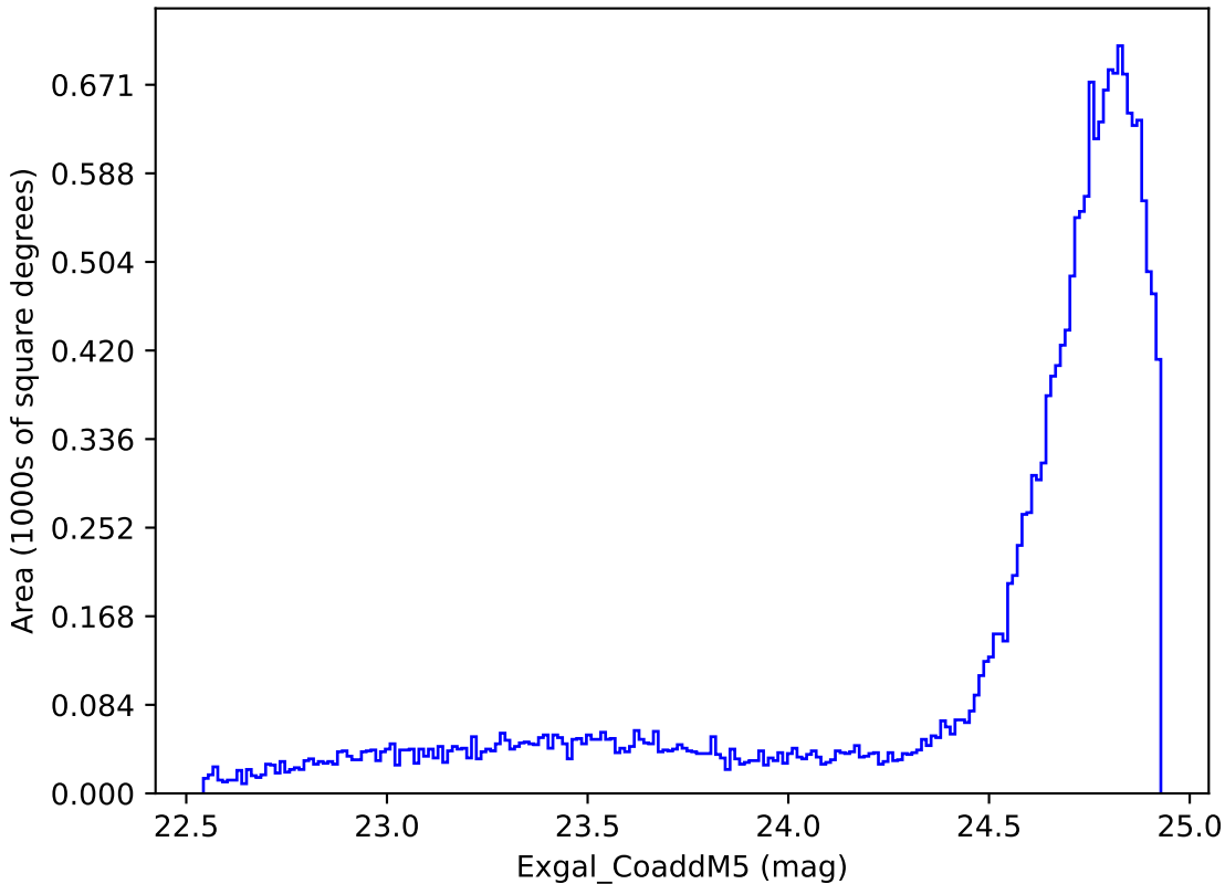
extra_ss_neo7_v3.4_10yrs All sky y band: Exgal_CoaddM5
