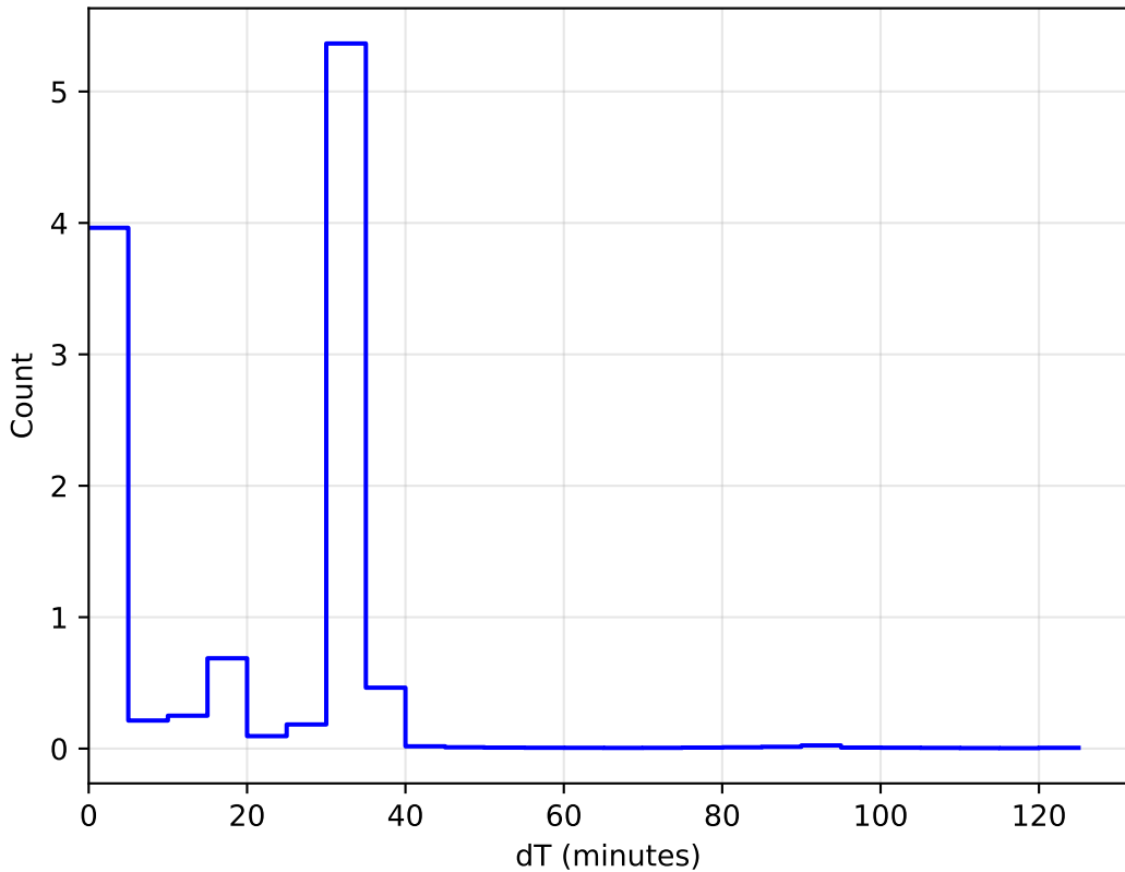
1e6 extra_ss_neo7_v3.4_10yrs WFD: DeltaT Histogram
