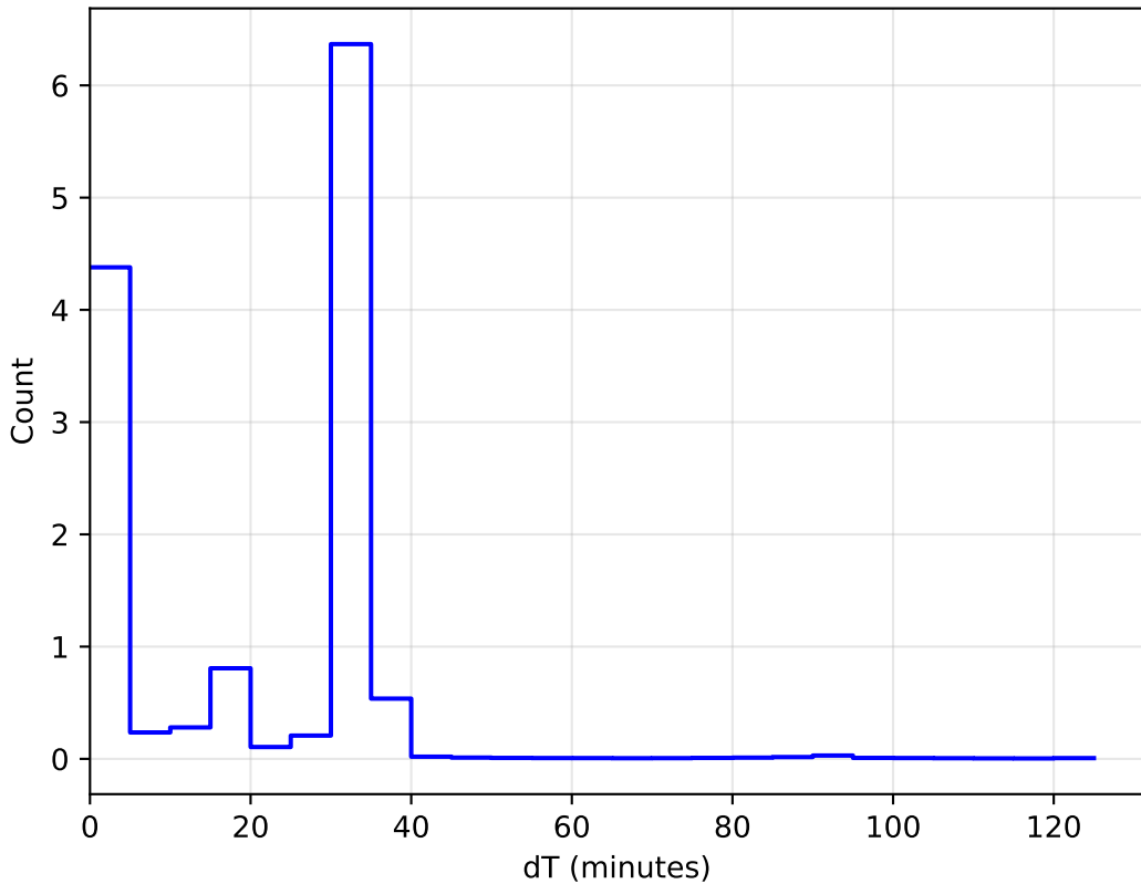
1e6 extra_ss_neo7_v3.4_10yrs All sky: DeltaT Histogram
