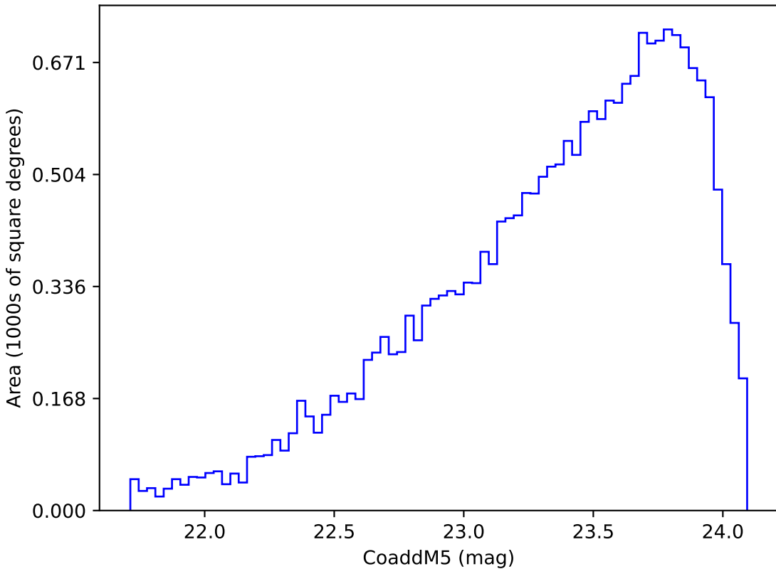
extra_ss_neo7_v3.4_10yrs Yr 3-4 y band: CoaddM5
