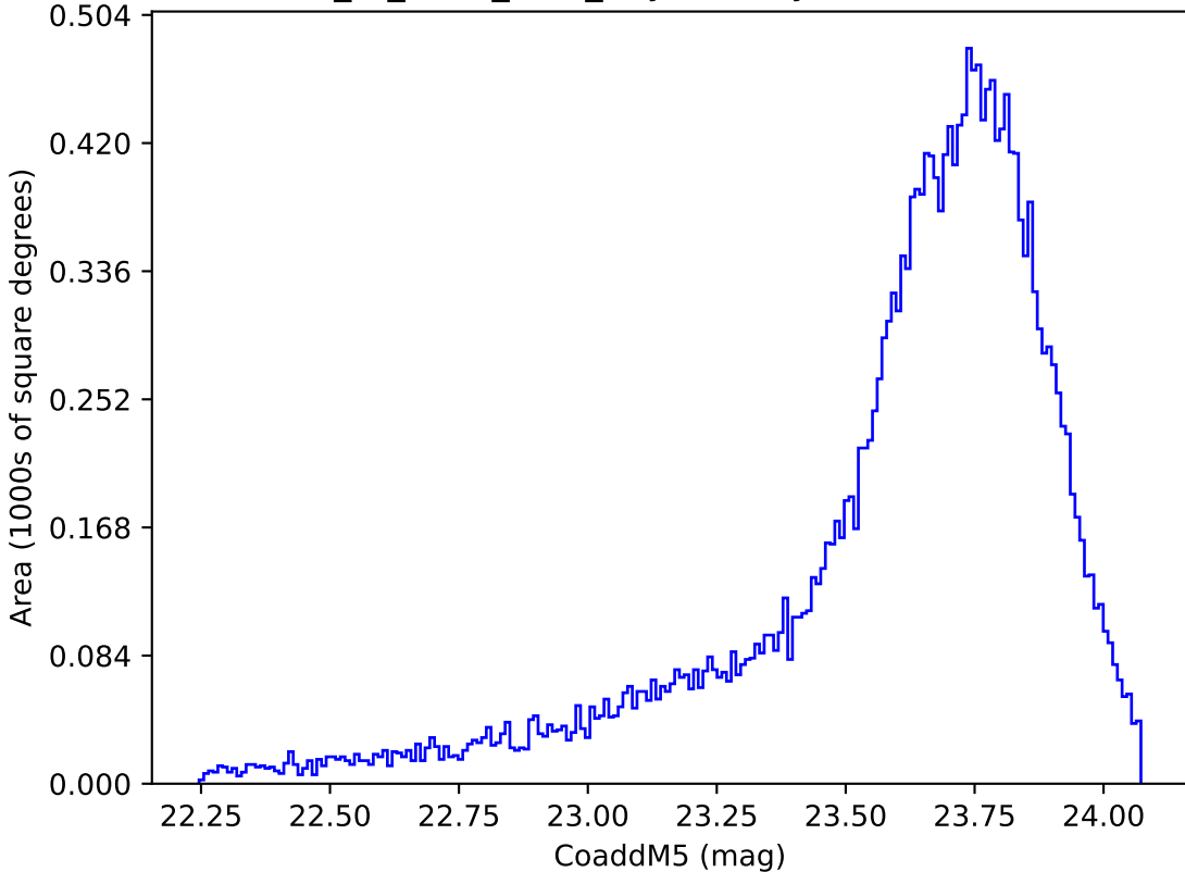
extra_ss_neo7_v3.4_10yrs Yr 1 y band: CoaddM5
