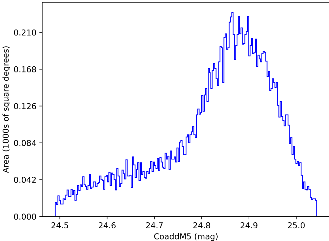
extra_ss_neo7_v3.4_10yrs WFD y band: CoaddM5
