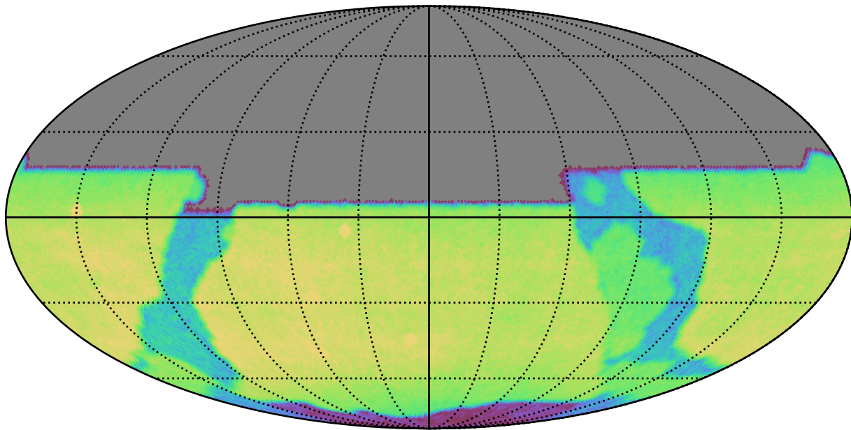
extra_ss_neo7_v3.4_10yrs All sky y band: CoaddM5
