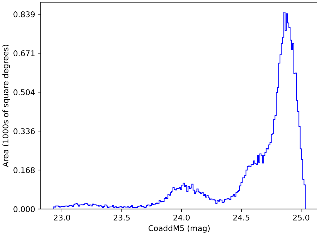
extra_ss_neo7_v3.4_10yrs All sky y band: CoaddM5
