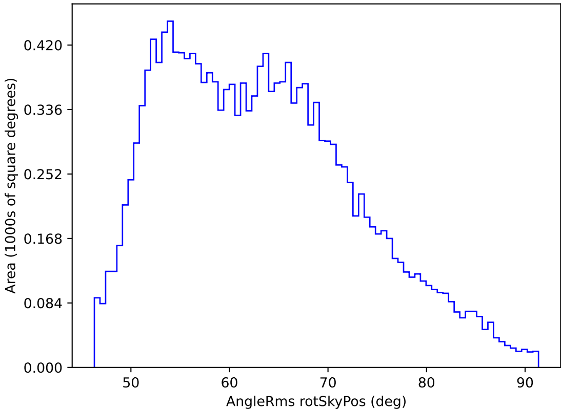
extra_ss_neo7_v3.4_10yrs WFD y band: AngleRms rotSkyPos
