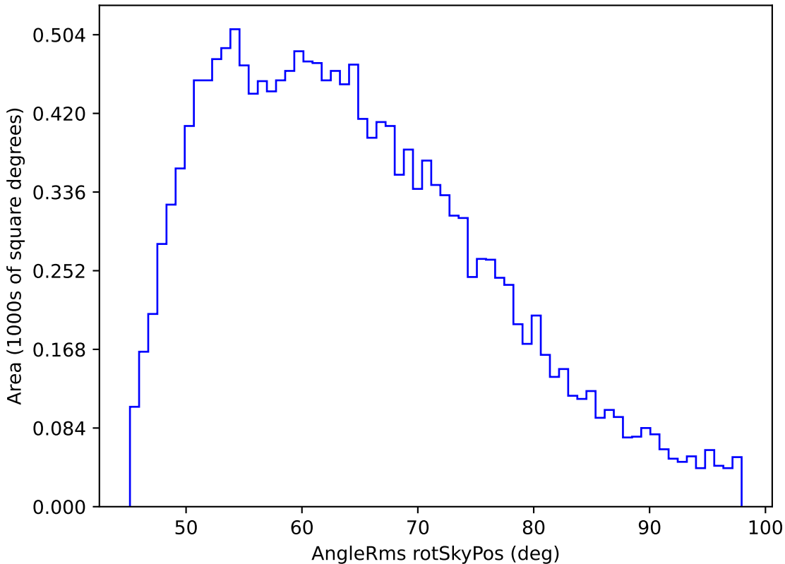
extra_ss_neo7_v3.4_10yrs WFD u band: AngleRms rotSkyPos
