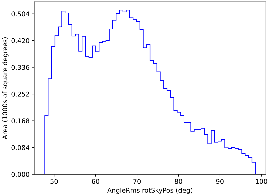
extra_ss_neo7_v3.4_10yrs WFD r band: AngleRms rotSkyPos
