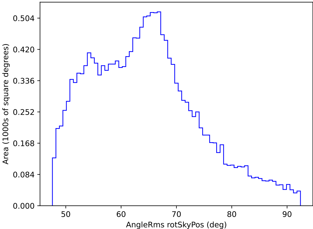
extra_ss_neo7_v3.4_10yrs WFD i band: AngleRms rotSkyPos
