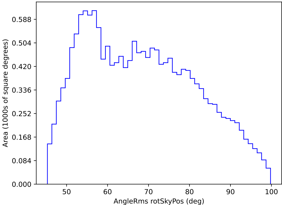
extra_ss_neo7_v3.4_10yrs WFD g band: AngleRms rotSkyPos
