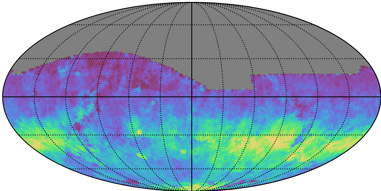
extra_ss_neo7_v3.4_10yrs All sky z band: AngleRms rotSkyPos
