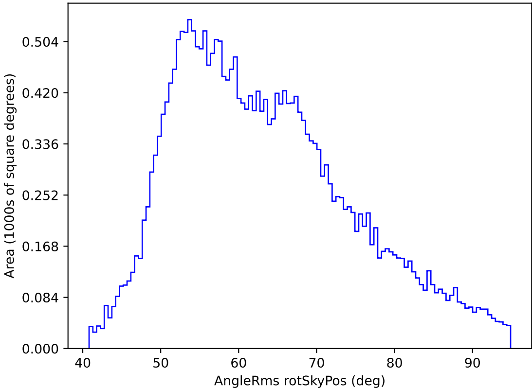
extra_ss_neo7_v3.4_10yrs All sky z band: AngleRms rotSkyPos
