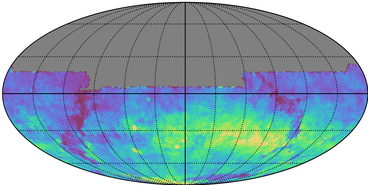
extra_ss_neo7_v3.4_10yrs All sky y band: AngleRms rotSkyPos
