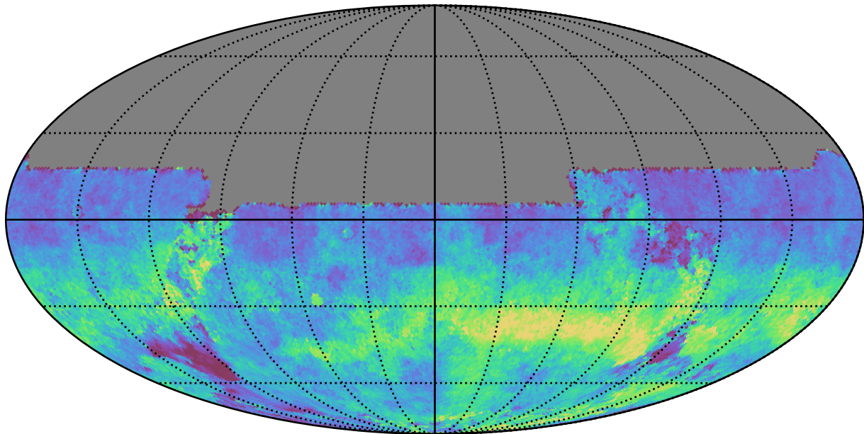
extra_ss_neo7_v3.4_10yrs All sky u band: AngleRms rotSkyPos
