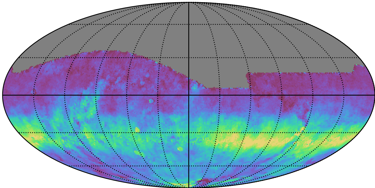
extra_ss_neo7_v3.4_10yrs All sky r band: AngleRms rotSkyPos
